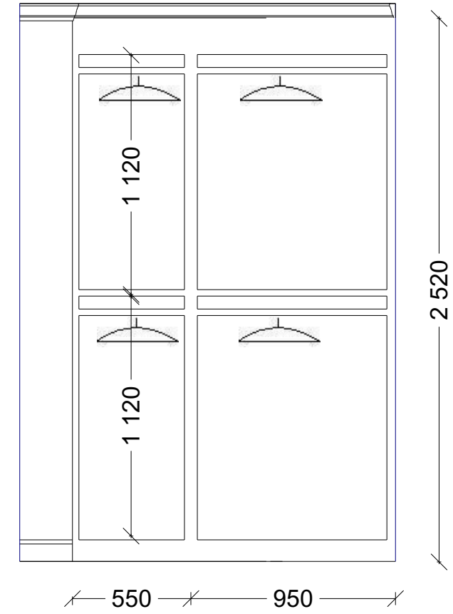
pohled C
