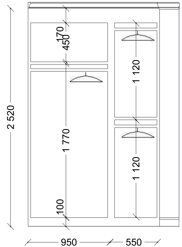
pohled C
