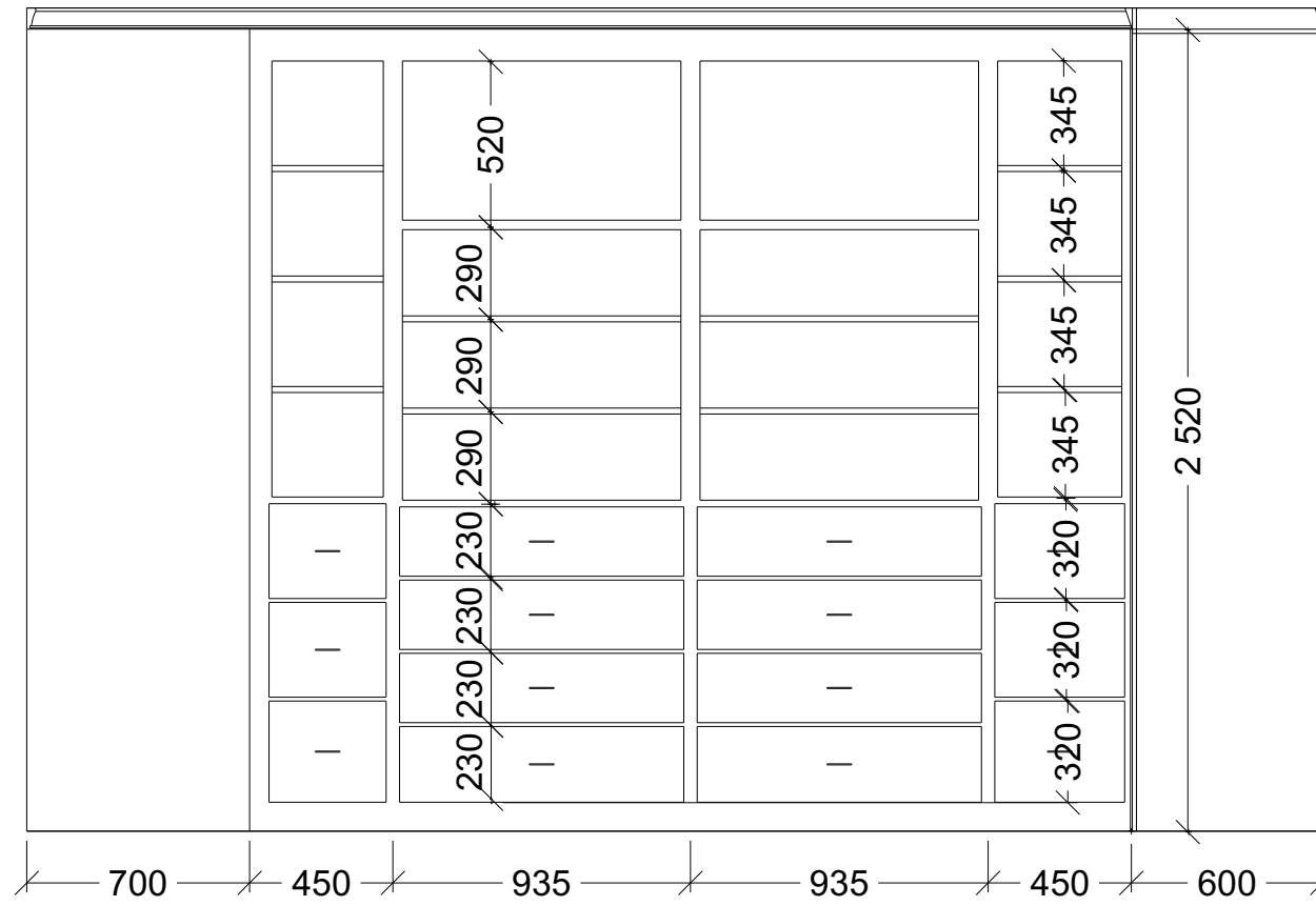
pohled A
